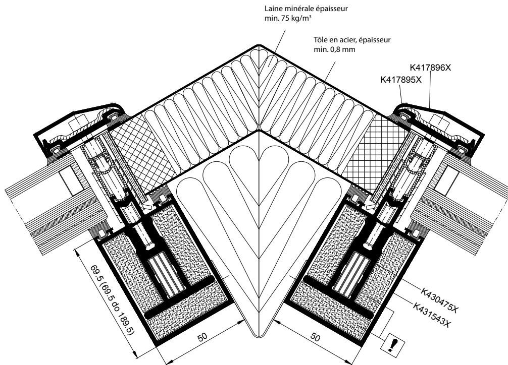
Assemblage : toit et mur-rideau, vue en coupe
