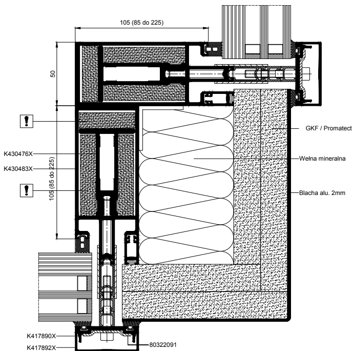
Montant 90o EI 30, vue en coupe
