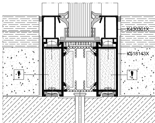
Cloison avec profilé intégré au sol, coupe transversale
