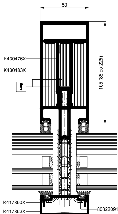
Montant EI 60, vue en coupe
