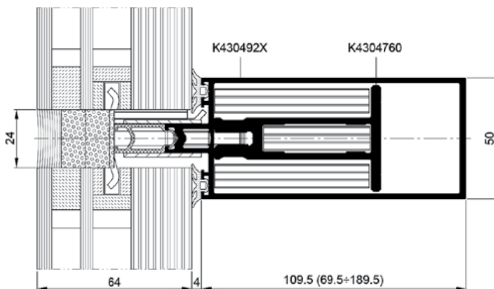
Traverse EI60 - coupe transversale
