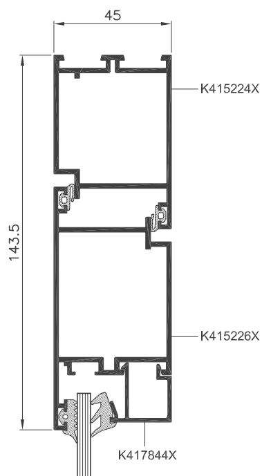
Dormant et vantail de porte – vue en coupe
