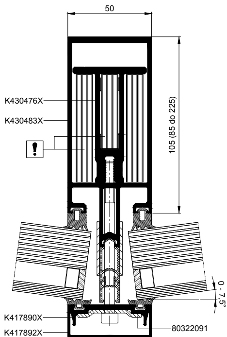
Montant +7,5° EI 60, vue en coupe
