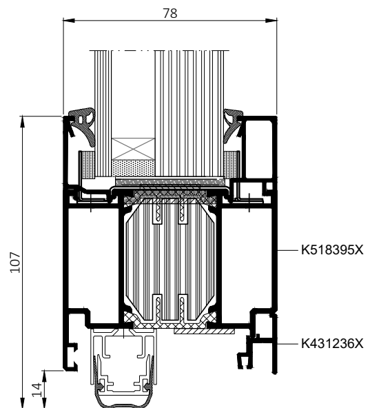
Dormant et vantail de porte joint « descendant » – vue en coupe
