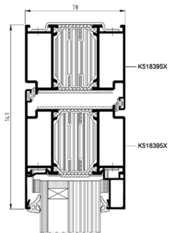
Dormant et vantail de porte avec inserts CI – vue en coupe
