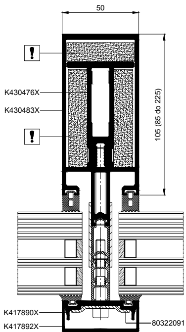
Montant EI 30, vue en coupe
