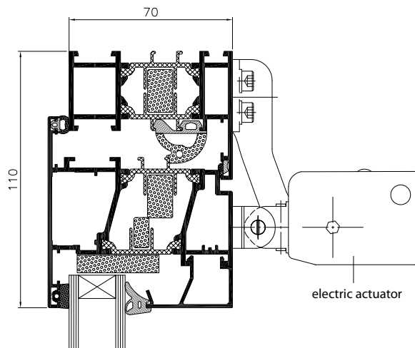
Fenêtre d'évacuation de fumées du système MB-70, vue en coupe
