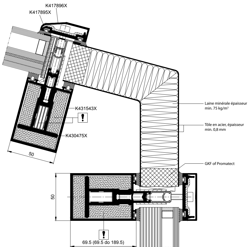
Assemblage : toit et mur-rideau, vue en coupe
