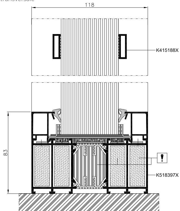
Cloison coupe-feu - coupe transversale
