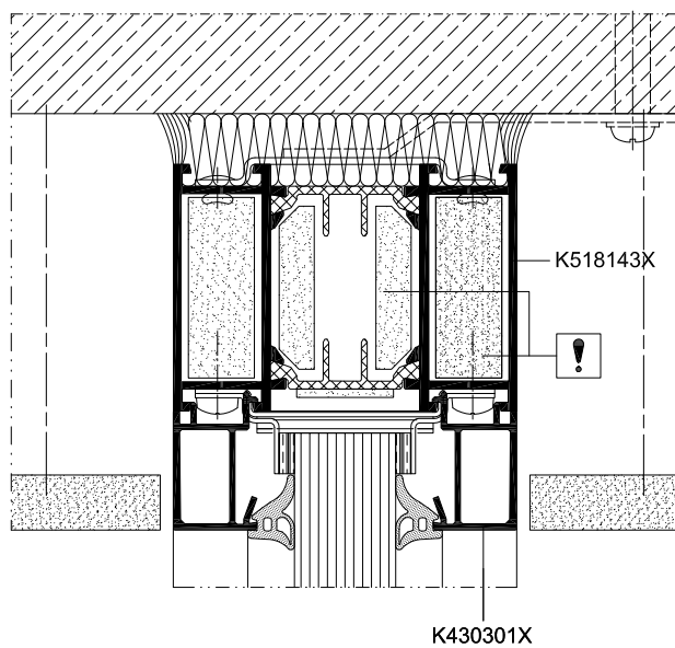
Cloison avec profilé intégré au plafond, coupe transversale
