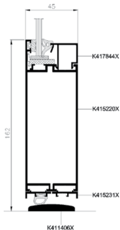
Porte avec seuil, coupe inférieure
