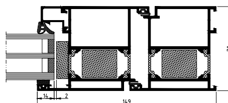
porte, vue en coupe
