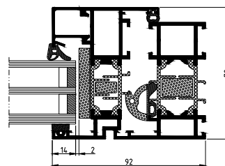
fenêtre, vue en coupe
